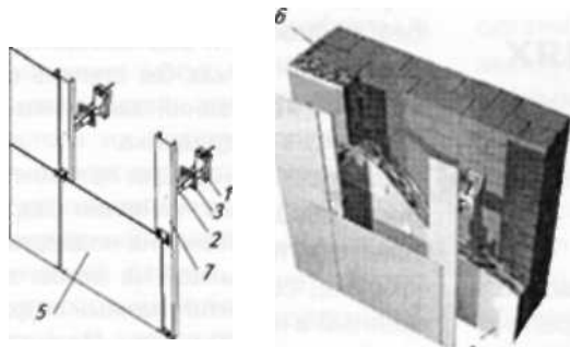
а – принципиальная схема; б – конструктивное решение; 1 – кронштейн; 2 – вставка; 3 – прижим утеплителя; 4 – утеплитель; 5 – облицовочная плита; 6 – кирпичная стена; 7 – профиль вертикальный
